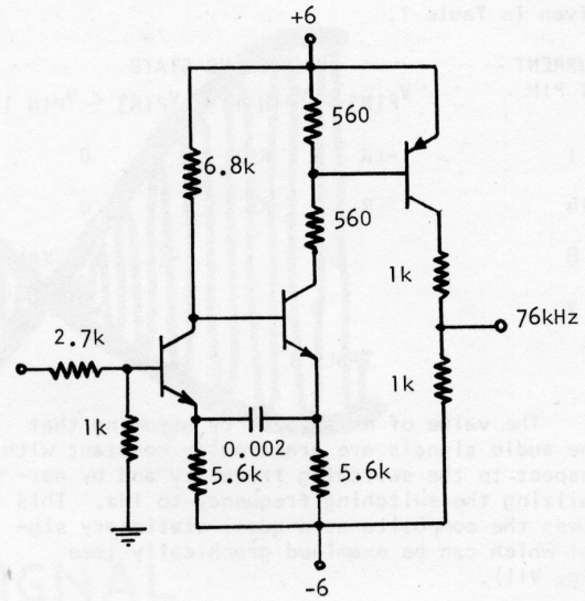
Fig. 5 76 kHz VCO
